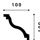
SL NOMASTYL® 100 x 100 x 2000 mm ART.NR. 3007251 EAN 5412938963527
