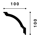
GP NOMASTYL® 100 x 100 x 2000 mm ART.NR. 3004245 EAN 5412938954631
