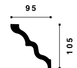
SM NOMASTYL® 105 x 95 x 2000 mm ART.NR. 3003179 EAN 5412938516853
