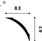
NE3 PURE NOMASTYL® 82 x 82 x 2000 mm ART.NR. 3015313 EAN 5412938974448
